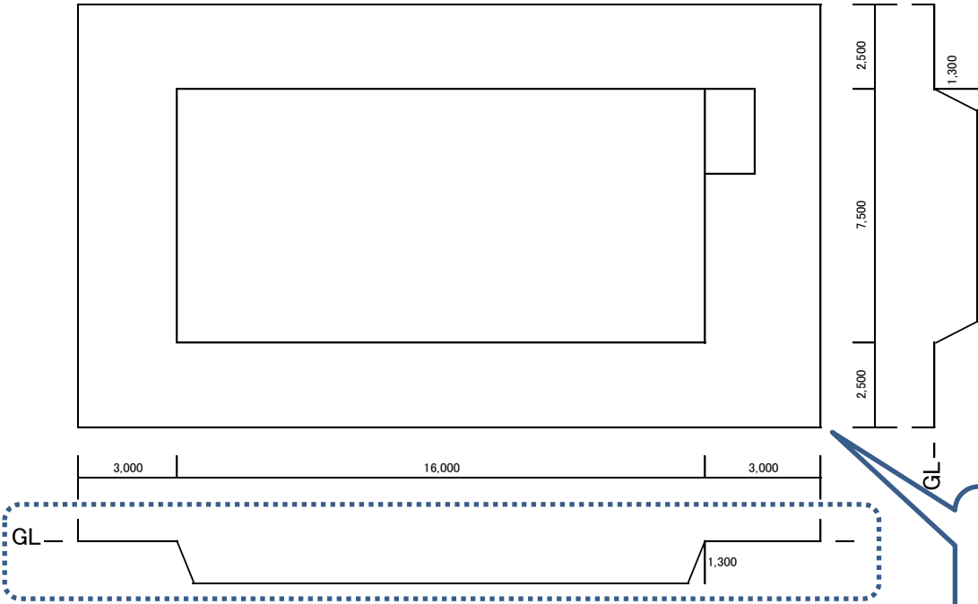
工事概略図 1/200
